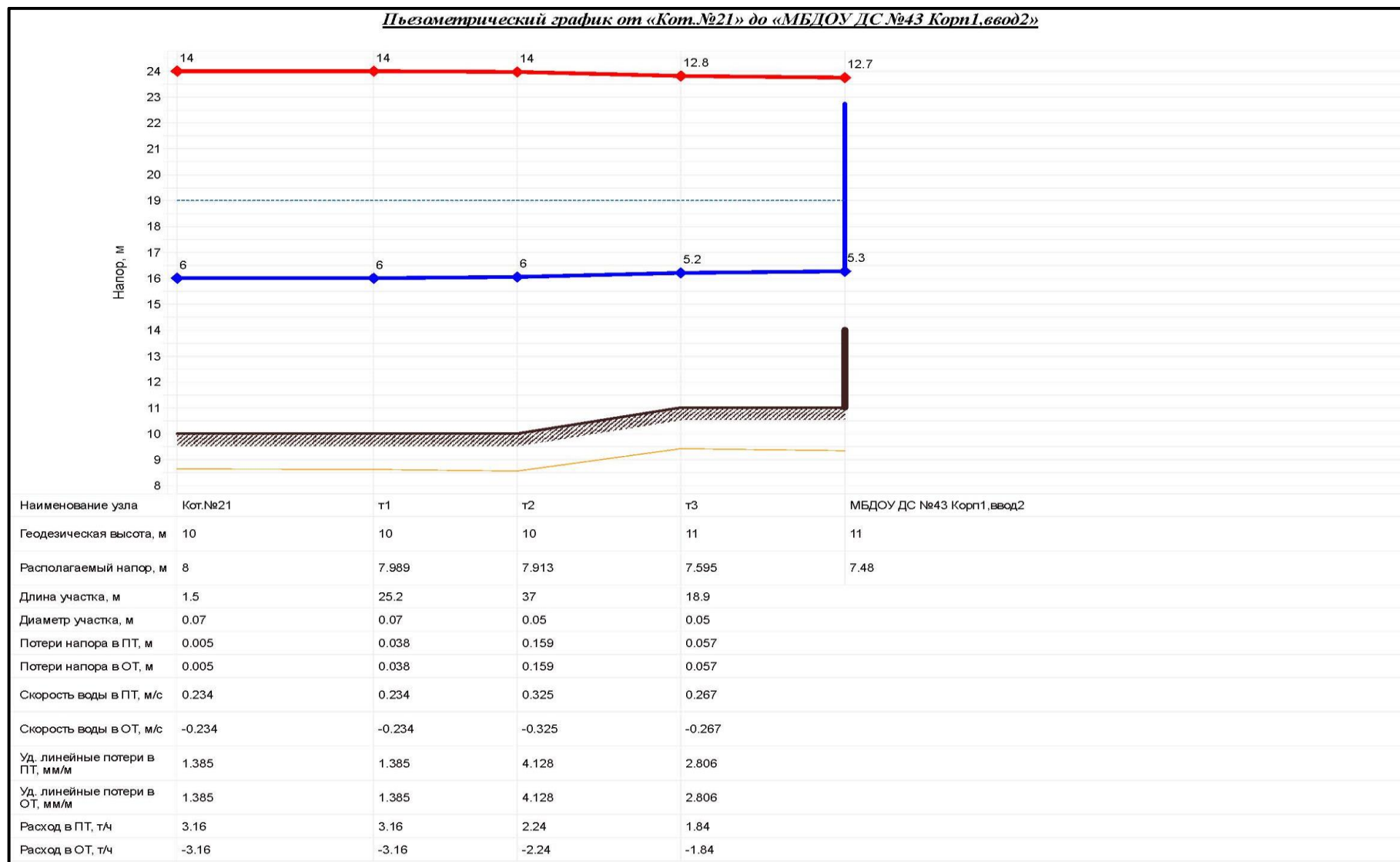
Рисунок 1.3.8.1 – Пьезометрический график Котельной №21, ст-ца Ахтанизовская (сущ. диаметры)
