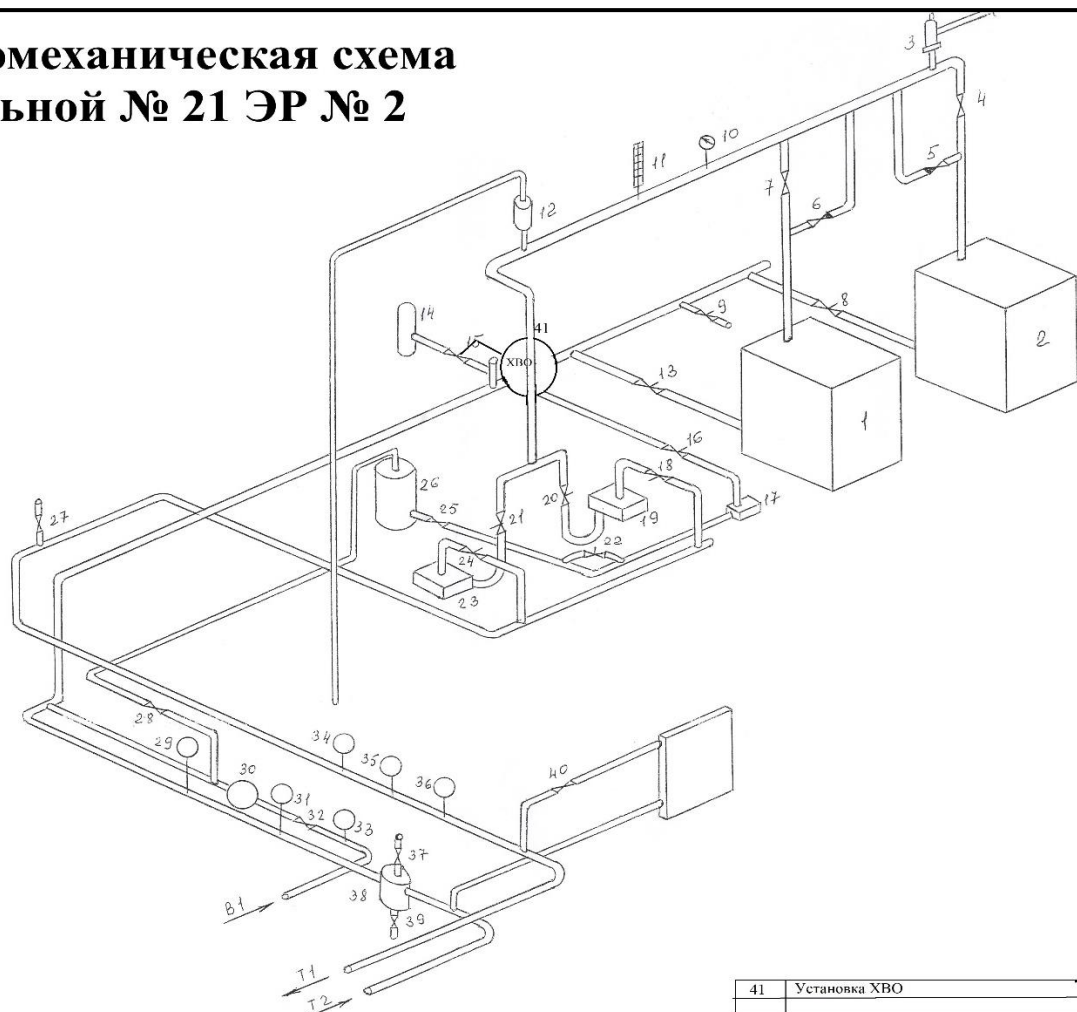
Рисунок 1.2.6.1 – Тепломеханическая схема котельной №21
