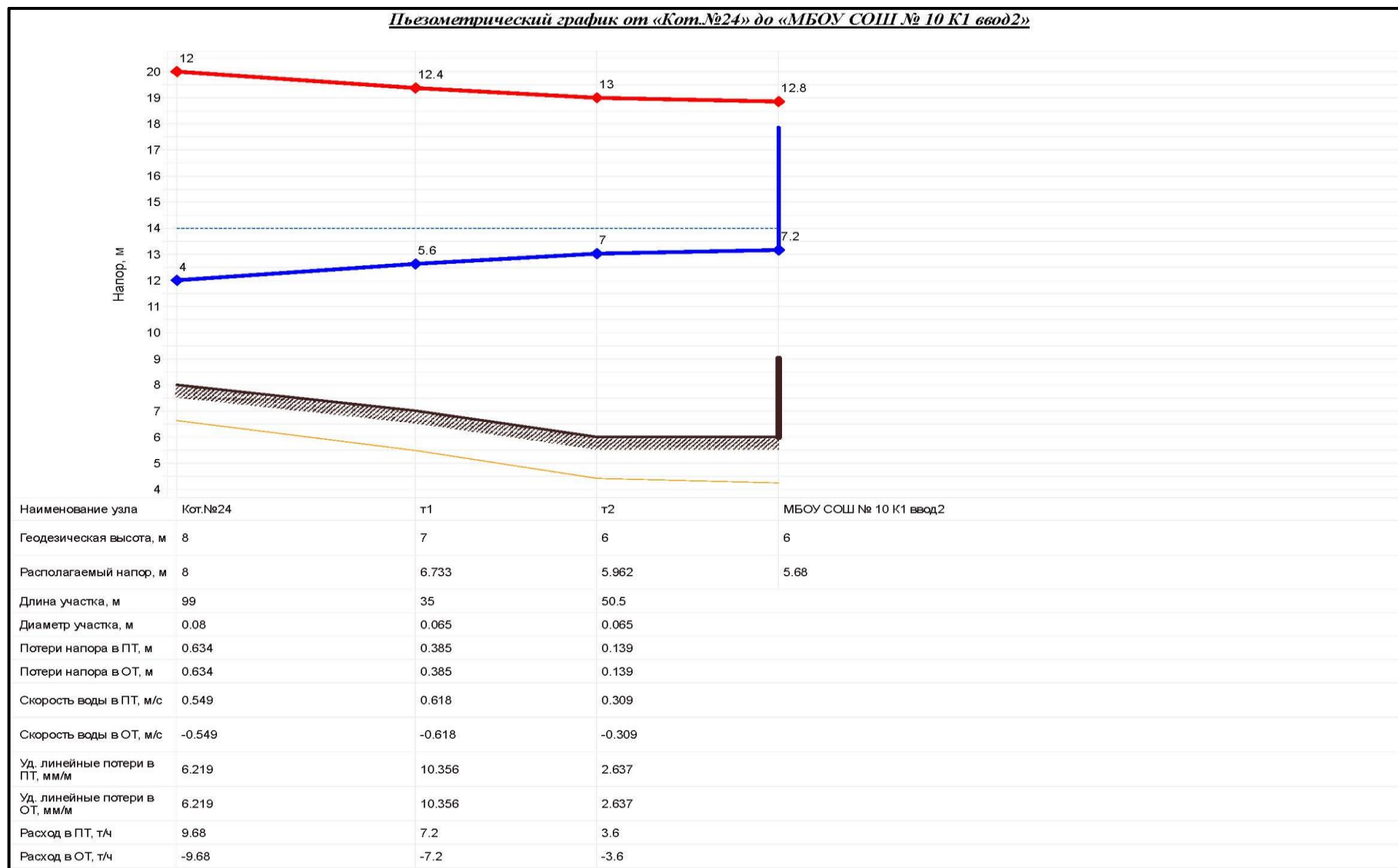
Рисунок 1.3.8.2 – Пьезометрический график Котельной №24, ст-ца Ахтанизовская
