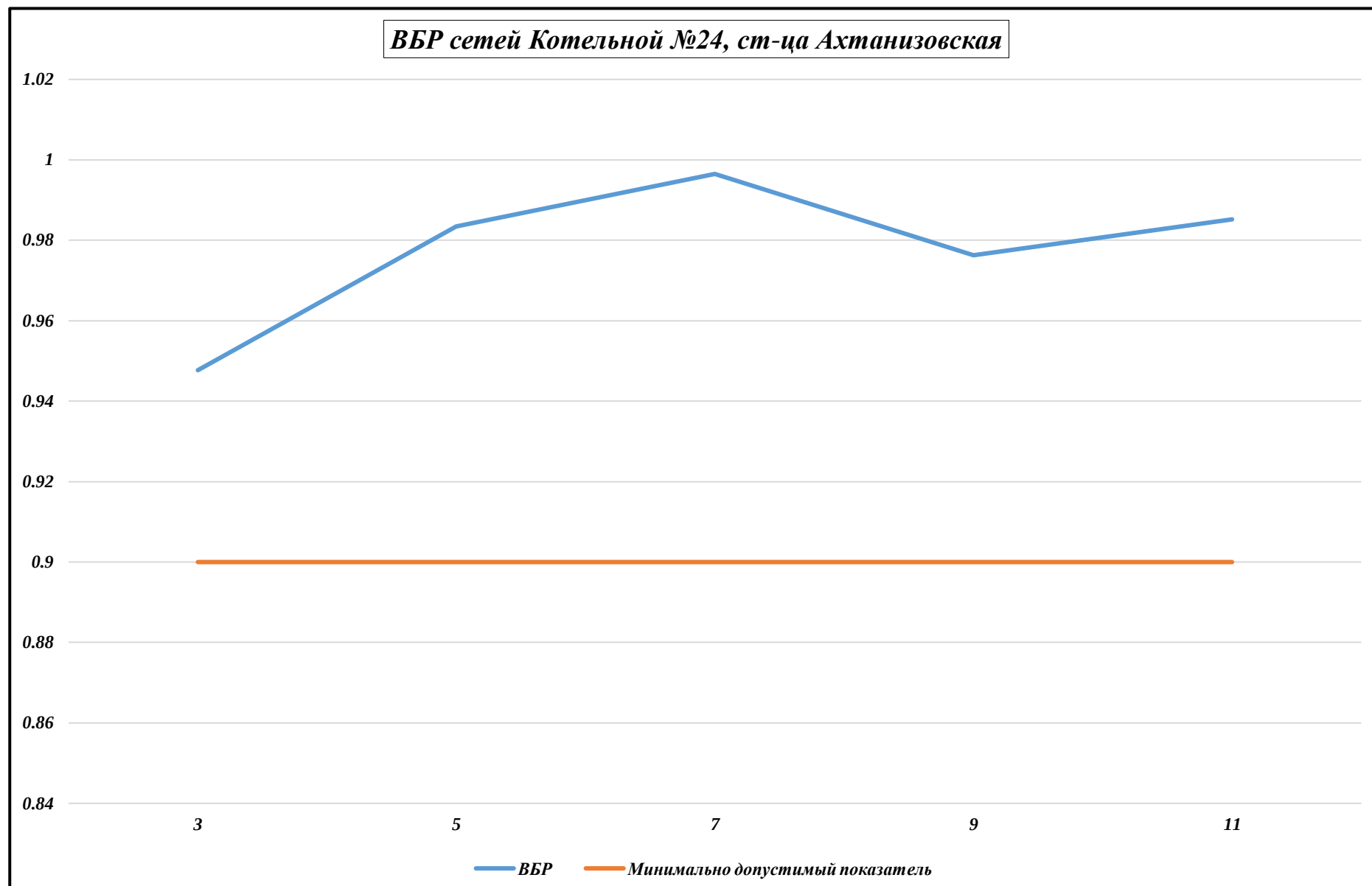
Рисунок 11.3.2 – ВБР Котельной №24, ст-ца Ахтанизовская
