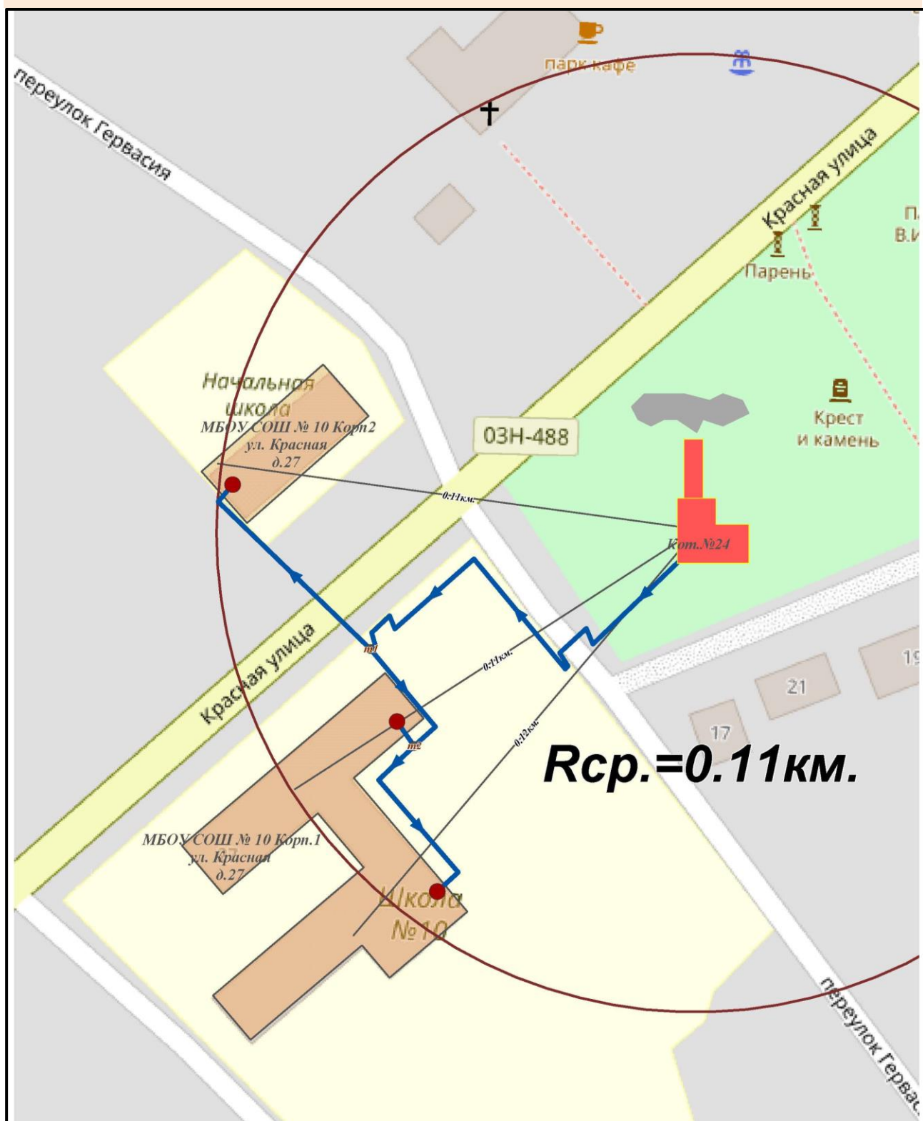
Рисунок 2.5.2 – РЭТС Котельной №24, ст-ца Ахтанизовская
