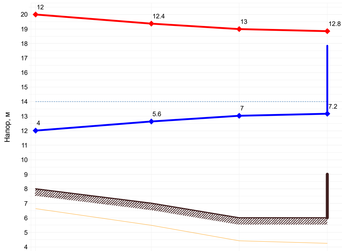
Пьезометрический график от «Кот.№24» до «МБОУ СОШ № 10 К1 ввод2»
